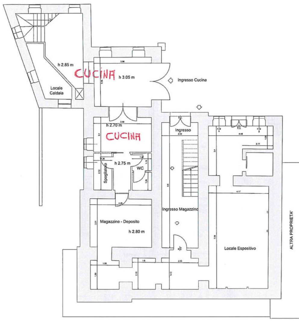
PIANTA PIANO SEMINTERRATO scala 1:50
