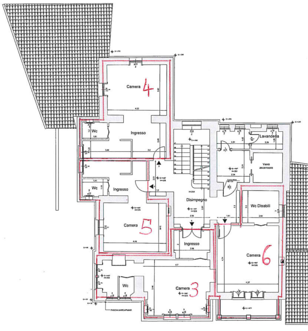
PIANTA PIANO SECONDO scala 1:50
